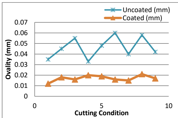
Fig. 7. Ovality
