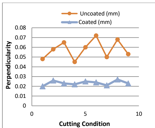
Fig. 8. Perpendicularity
